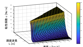
ダンパの設置値マップ
