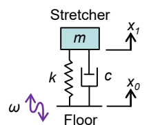
防振台の簡易モデル
